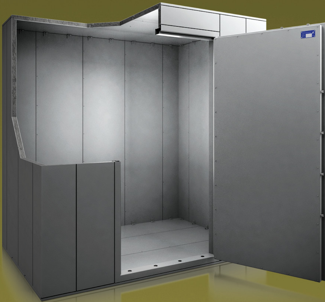
Abbildung: Modellversion Waffenraum Klasse 1 / I nach EN 1143-1 im Anschnitt
